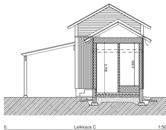
Luonnos, Leikkaus:
