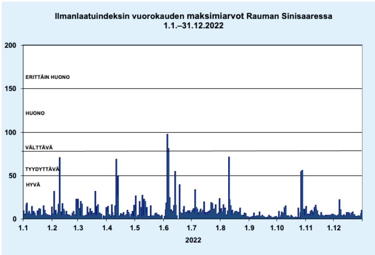
Kuva 5. Vuorokauden suurimmat ilmanlaatuindeksin arvot Rauman Sinisaarella vuonna 2022.
