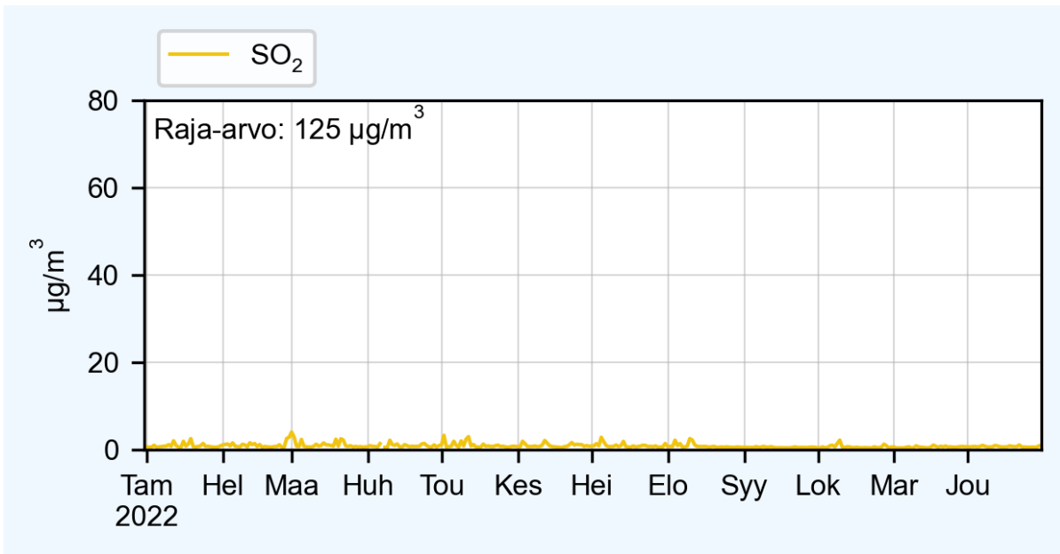
Kuva 3. Rikkidioksidin ( \text{SO}_2 ) vuorokausipitoisuudet ( \mu\text{g}/\text{m}^3 ) Rauman sinisaarella vuonna 2022.
