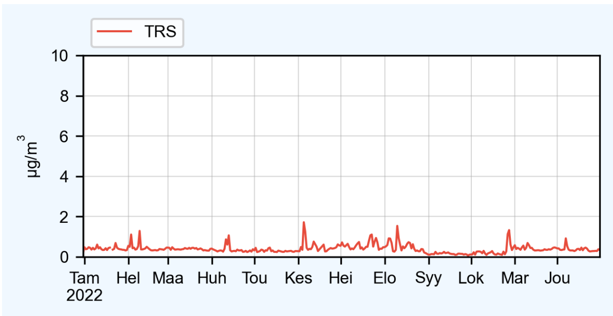
Kuva 4. Haisevien rikkiyhdisteiden (TRS) vuorokausipitoisuudet ( \mu\text{g}(\text{S})/\text{m}^3 ) Rauman sinisaarella vuonna 2022.
