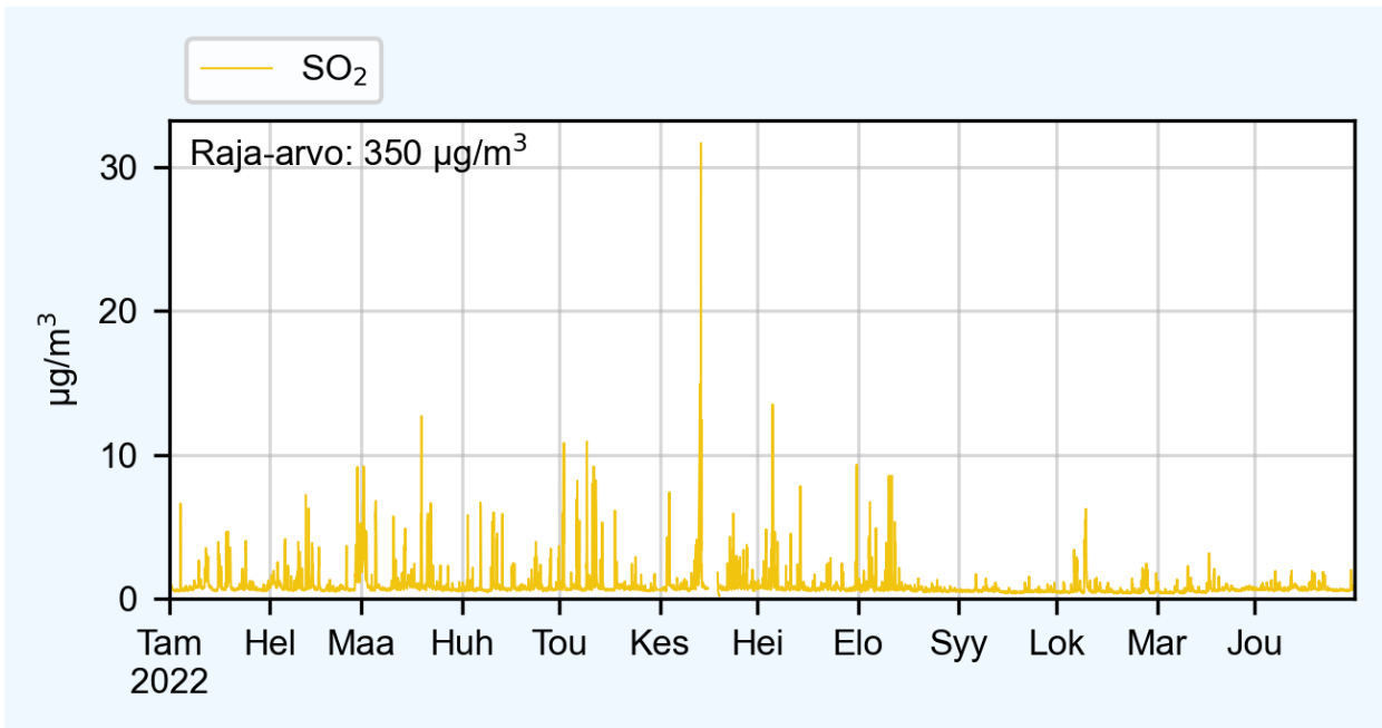
Kuva 1. Rikkidioksidin (SO 2 ) tuntipitoisuudet (µg/m 3 ) Rauman sinisaarella vuonna 2022.
