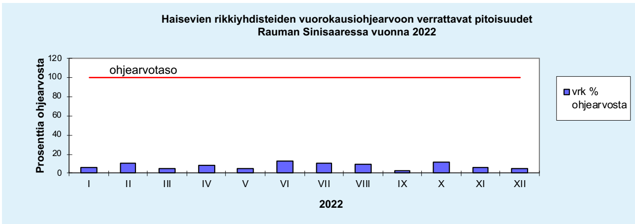
Kuva 1. Haisevien rikkiyhdisteiden vuorokausiohjearvoon verrattavat pitoisuudet.
