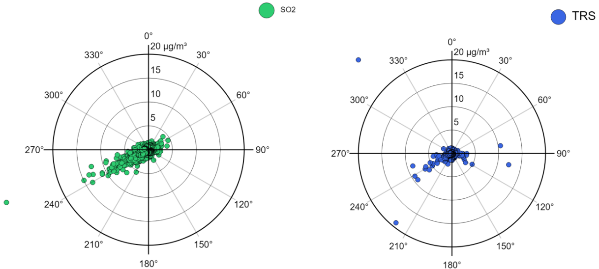
Kuva 9. Rauman Sinisaaren mittasasemalla mitatut SO 2 :n ja TRS:n pitoisuudet tuulensuunnittain mittausjaksolla 1.1.–31.12.2022.
