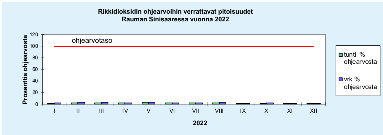
Kuva 6. Rikkidioksidin ohjearvopitoisuudet Sinisaarella 2022.
