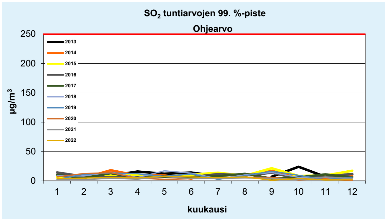
Kuva 10. Rikkidioksidin tuntiohjearvoon (250 µg/m 3 ) verrannolliset pitoisuudet Rauman Sinisaassa vuosina 2013–2022.
