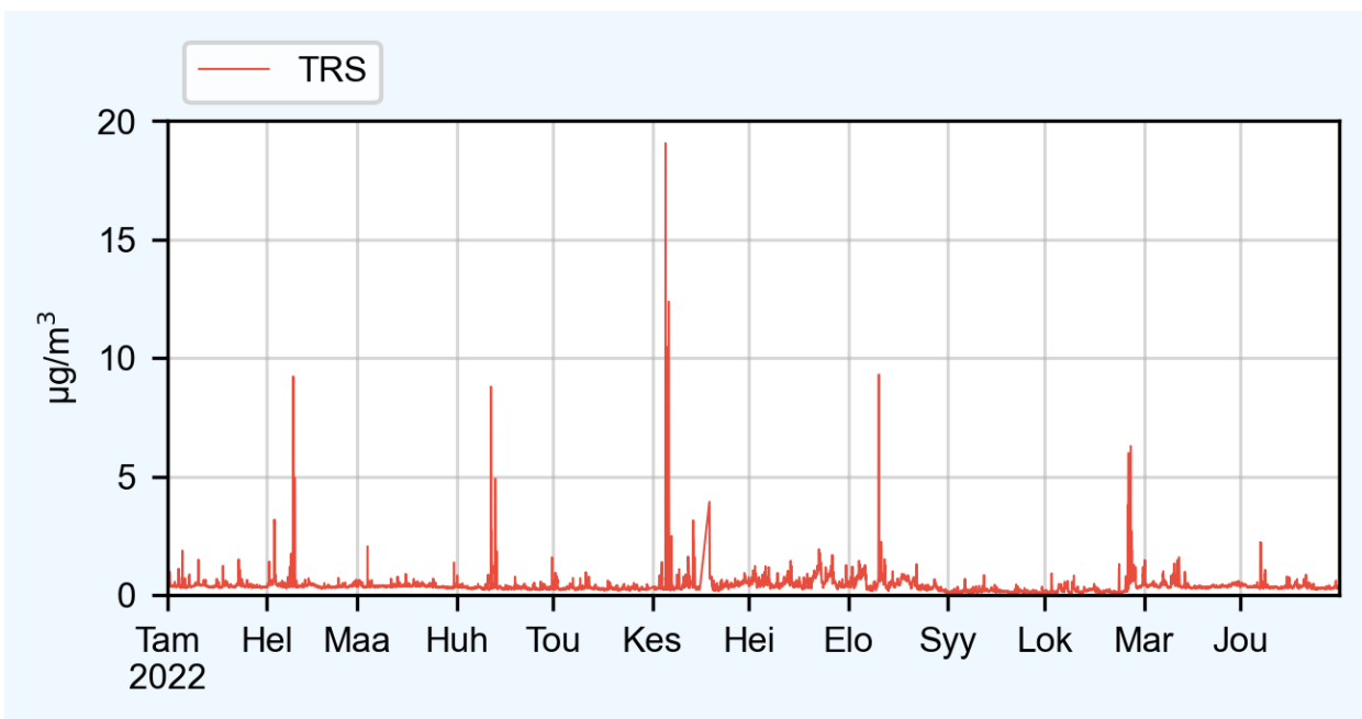
Kuva 2. Haisevien rikkiyhdisteiden (TRS) tuntipitoisuudet (µg(S)/m 3 ) Rauman sinisaarella vuonna 2022.
