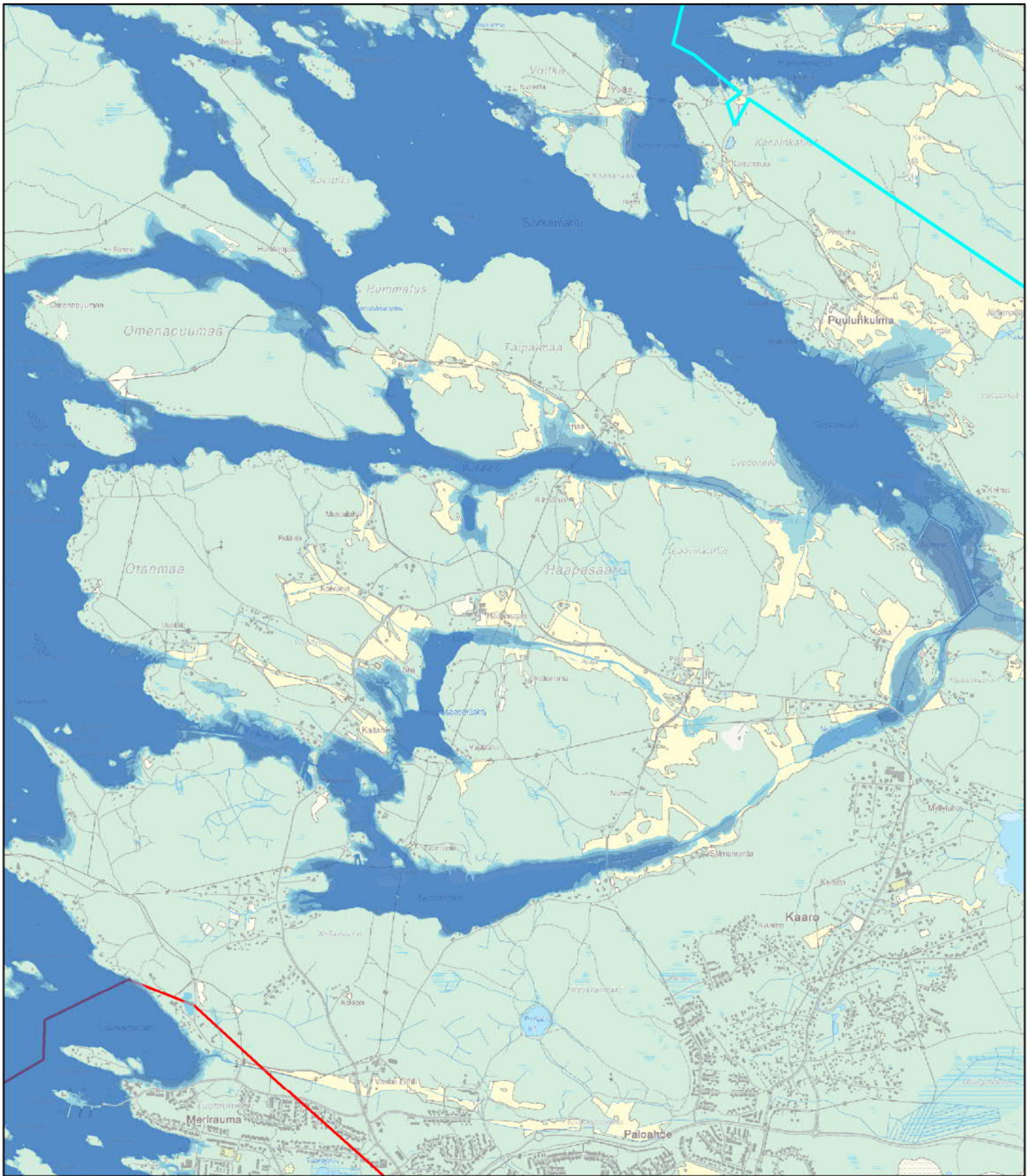
Rauma pohjoineni 1/250a vedenkorkeus 1,728 m (N2000)
